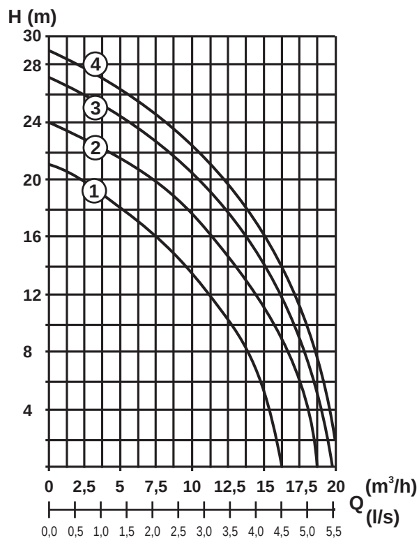
Rysunek 1: Budowa i charakterystyka hydrauliczna pompy serii WIR-R
