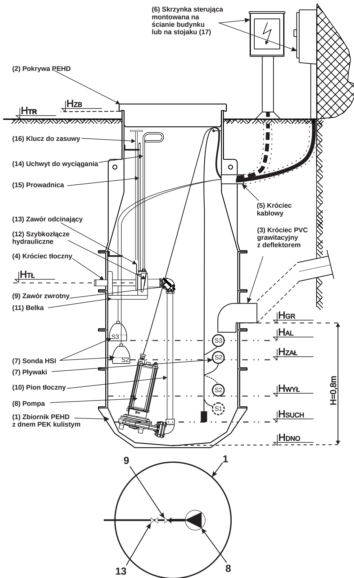
Rysunek 3: Kompaktowa pompownia INWAP z pompą WIR
