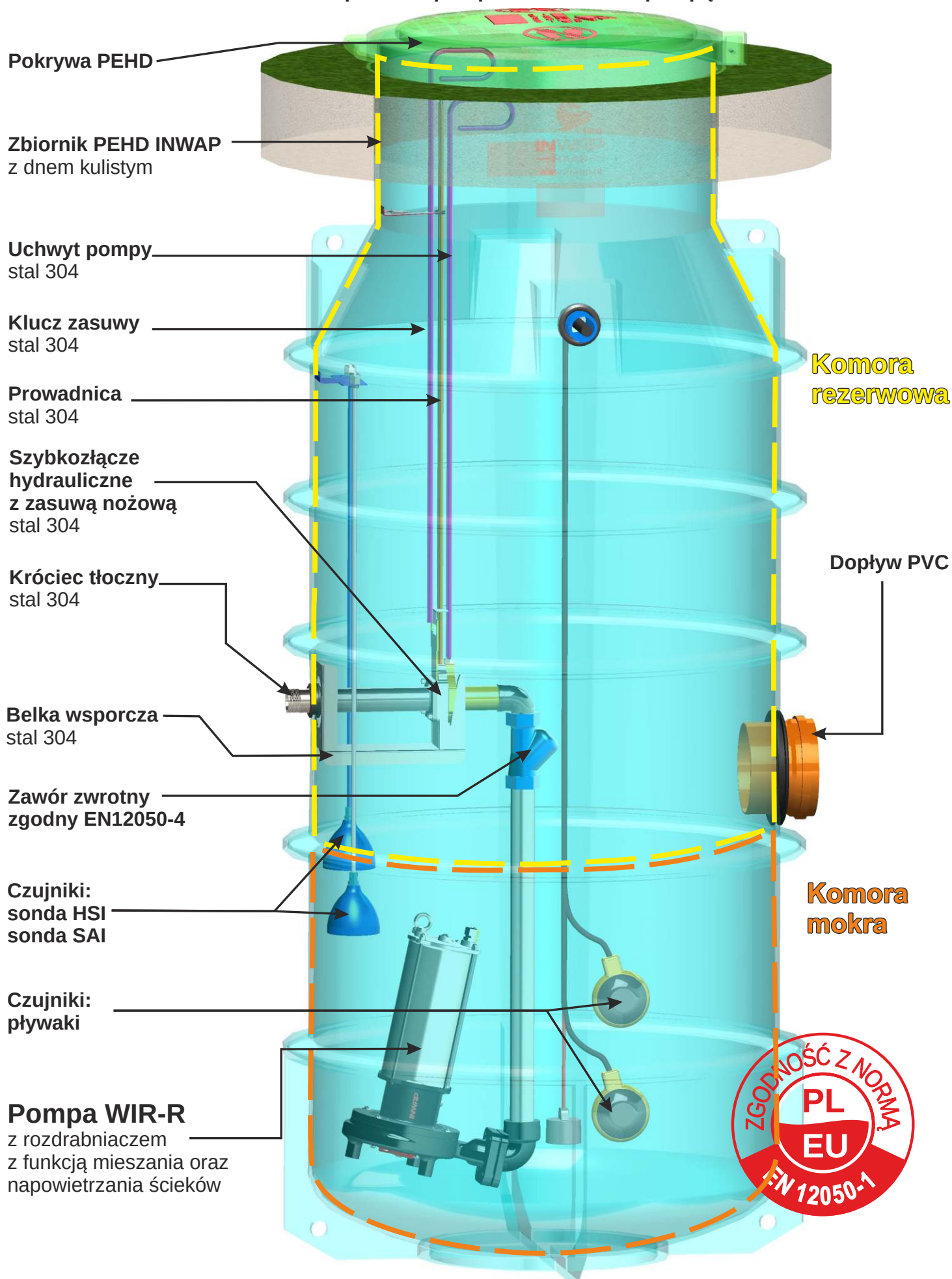
RYSUNEK 3: Kompaktowa pompownia INWAP z pompą WIR-R
